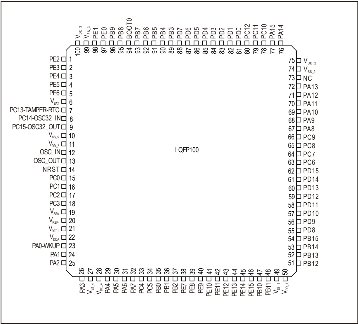
图 5-2 LQFP100 引脚分布
