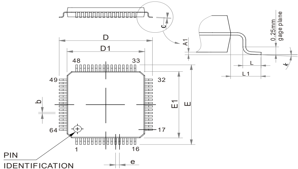
图 6-5 LQFP64 封装图
