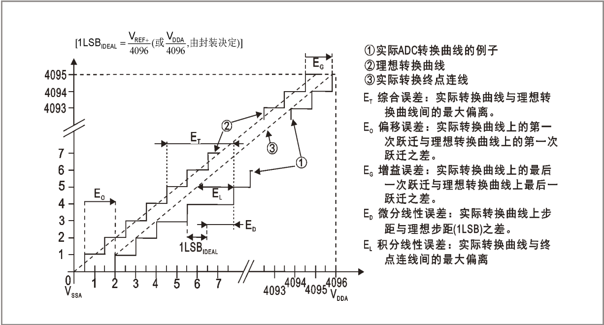
图 4-11 ADC 精度特性
