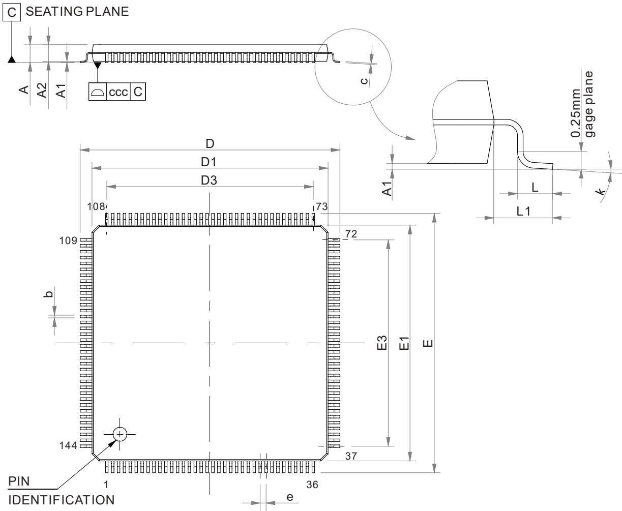
图 6-1 LQFP144 封装图
