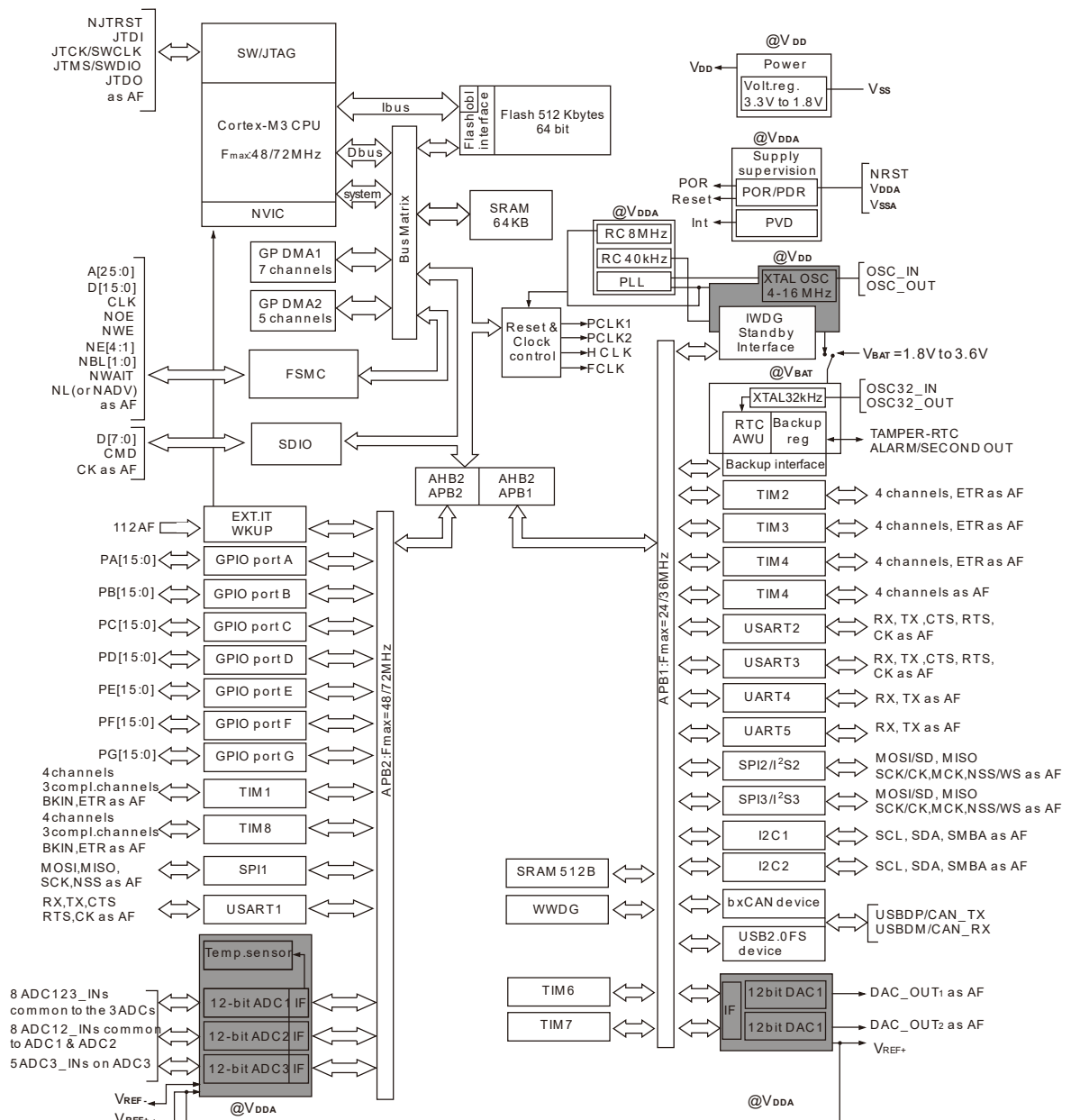
图 3-1 LTM32F103 系列芯片功能框图
