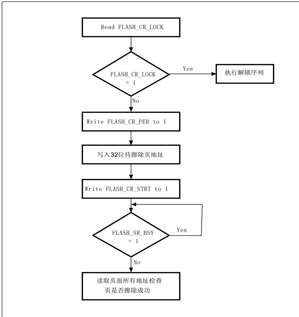
图 2-2 页面擦除
