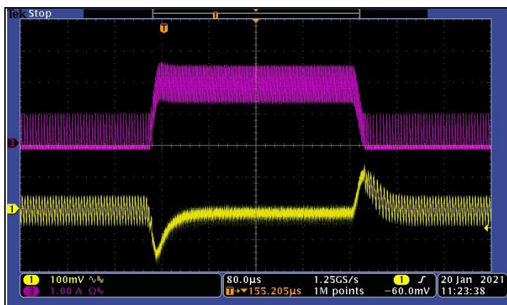
图 7 负载瞬态响应 ( V_{in}=12V , V_{out}=3.3V , I_{LOAD}=0.2-2A )
