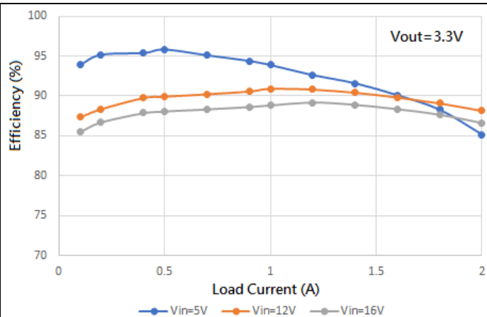
图 2 效率与负载
