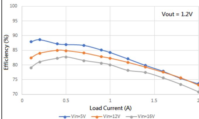
图 3 效率与负载
