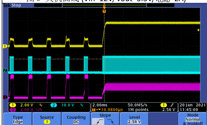
图 9 关机曲线 ( V_{in}=12V , V_{out}=3.3V , I_{LOAD}=2A )
