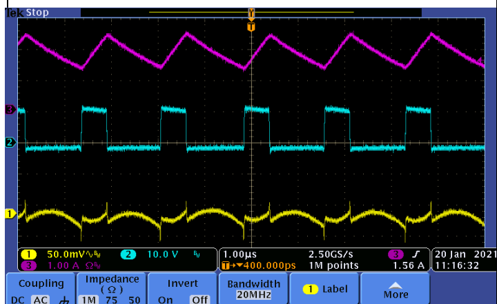
图 4 输出纹波 ( V_{IN}=12V , V_{OUT}=3.3V , I_{LOAD}=2A )
