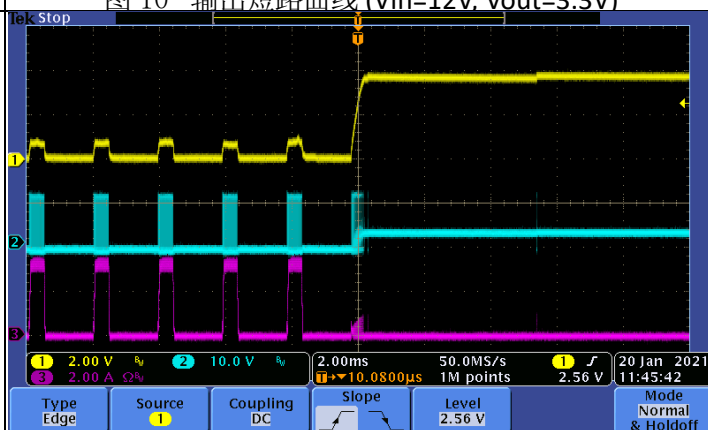
图 10 输出短路曲线 ( V_{in}=12V , V_{out}=3.3V )
