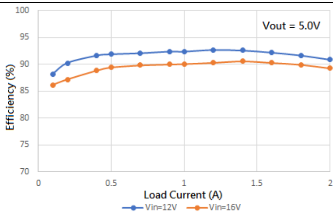
图 1 效率与负载
