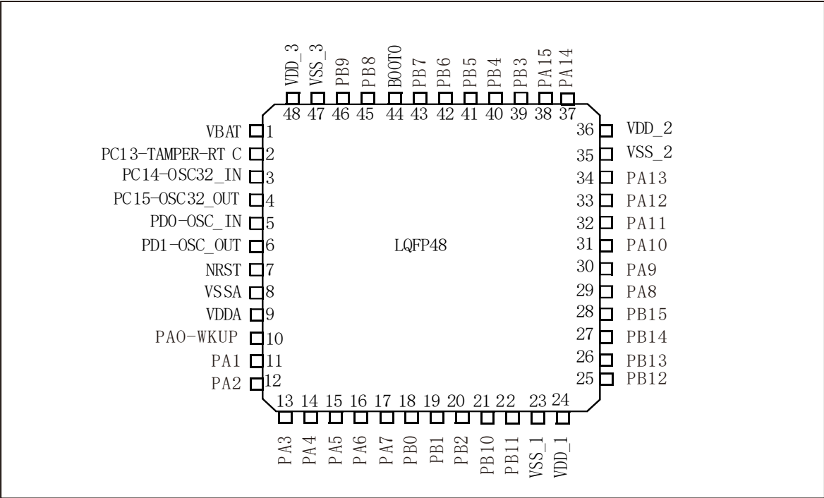
图 5-4 LQFP48 引脚分布
