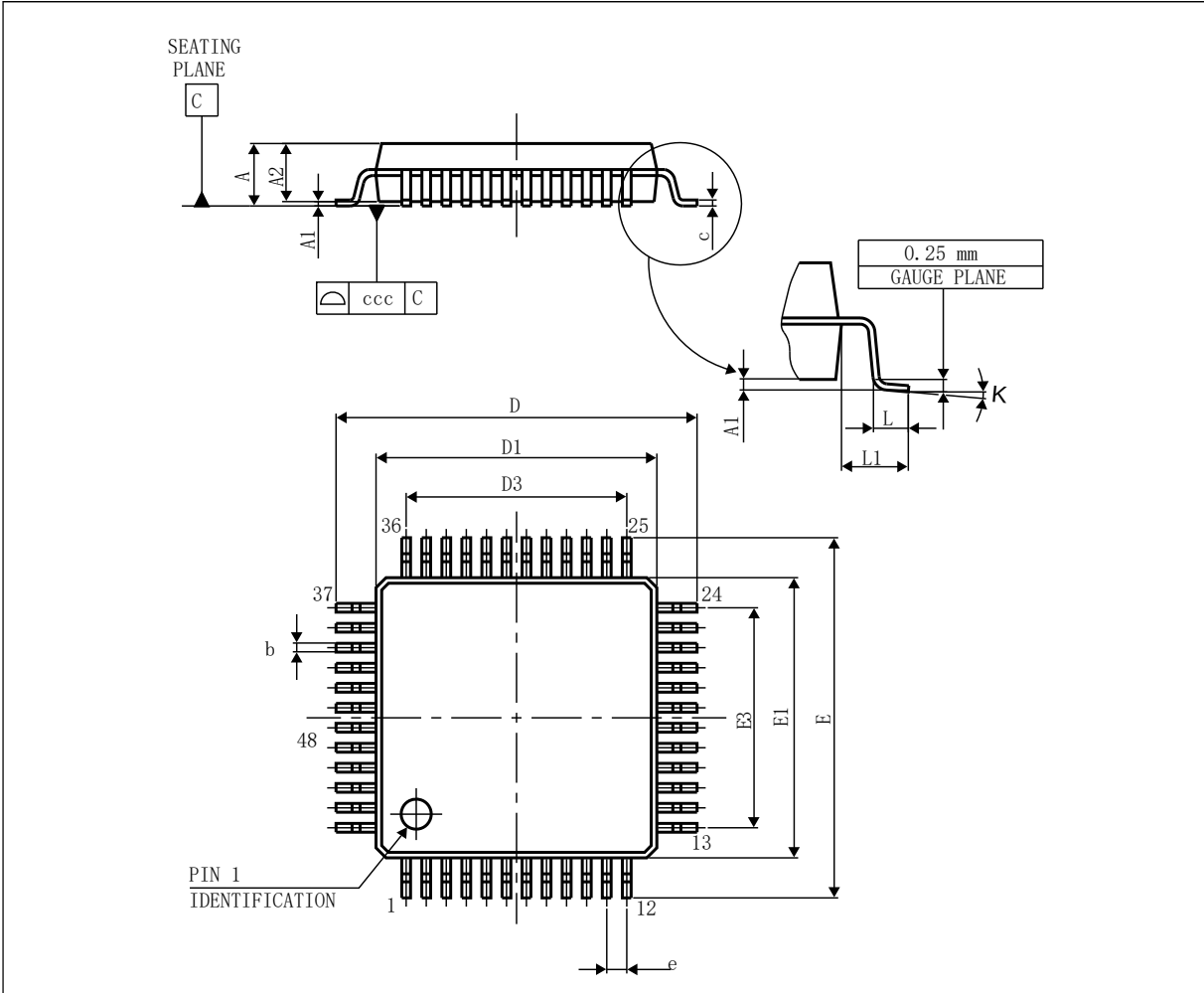
图 6-7 LQFP48 封装图
