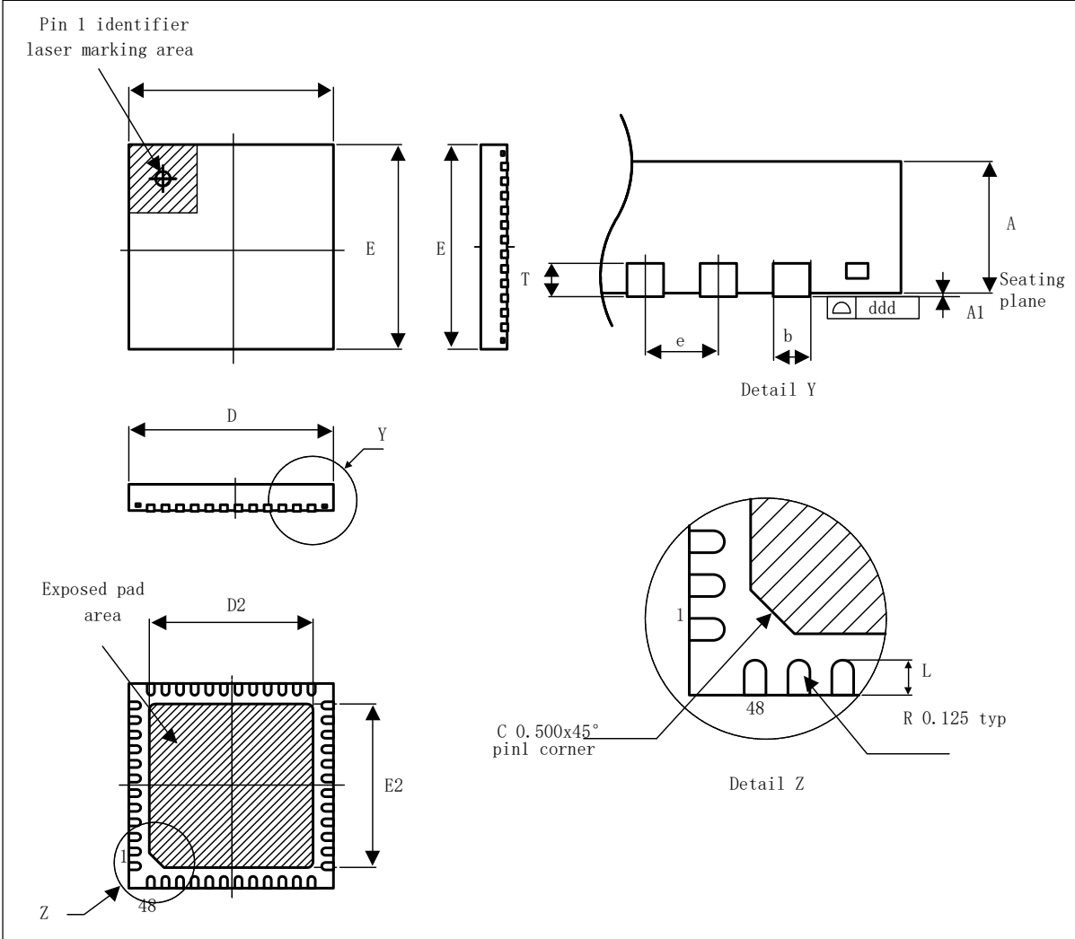
图 6-9 QFN48 封装图
