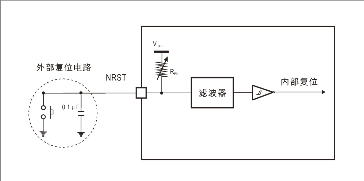
图 4-1 外部复位电路图
