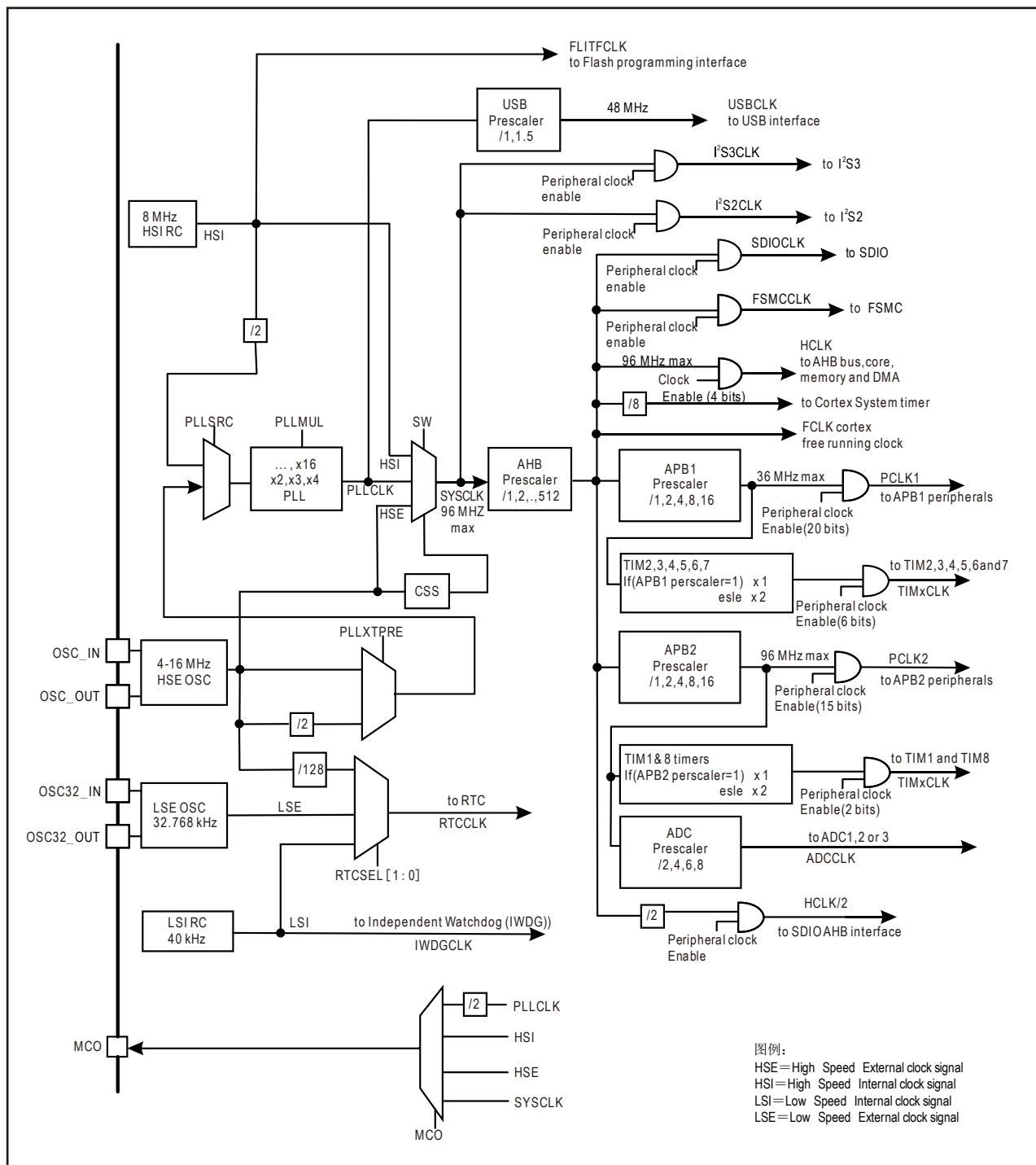
图 3-2 LTM32F103 系列芯片时钟树
