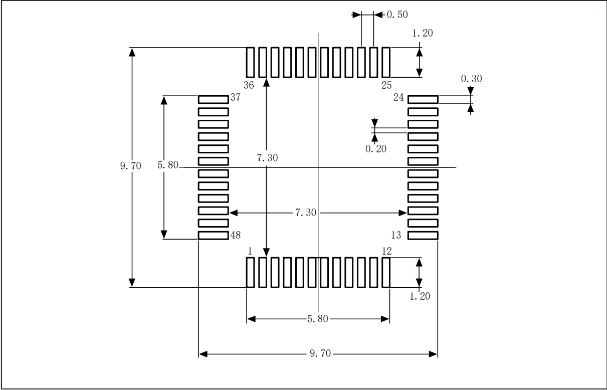
LQFP48 封装芯片的 PCB 推荐安装尺寸:
