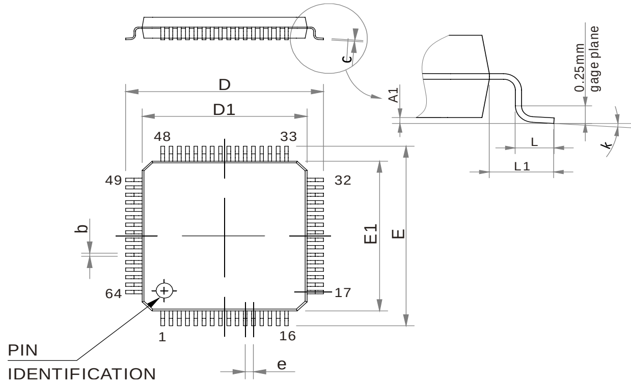
图 6-5 LQFP64 封装图
