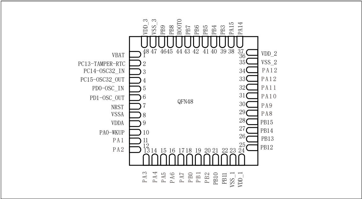
图 5-5 QFN48 引脚分布
