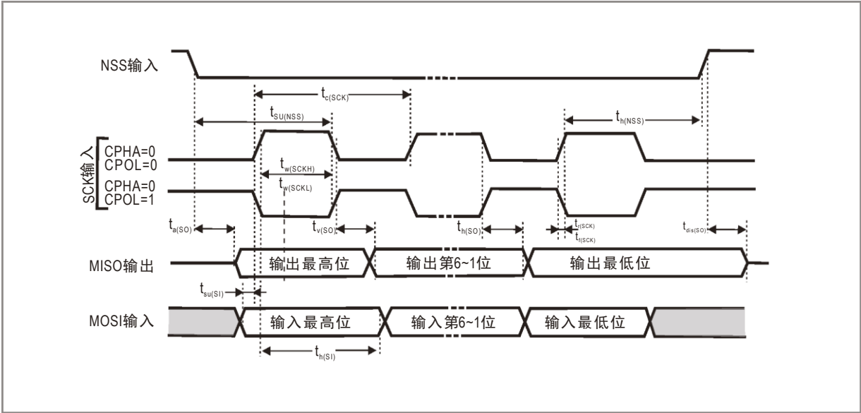
图 4-3 SPI 从模式时序图 (第一个边沿采样)
