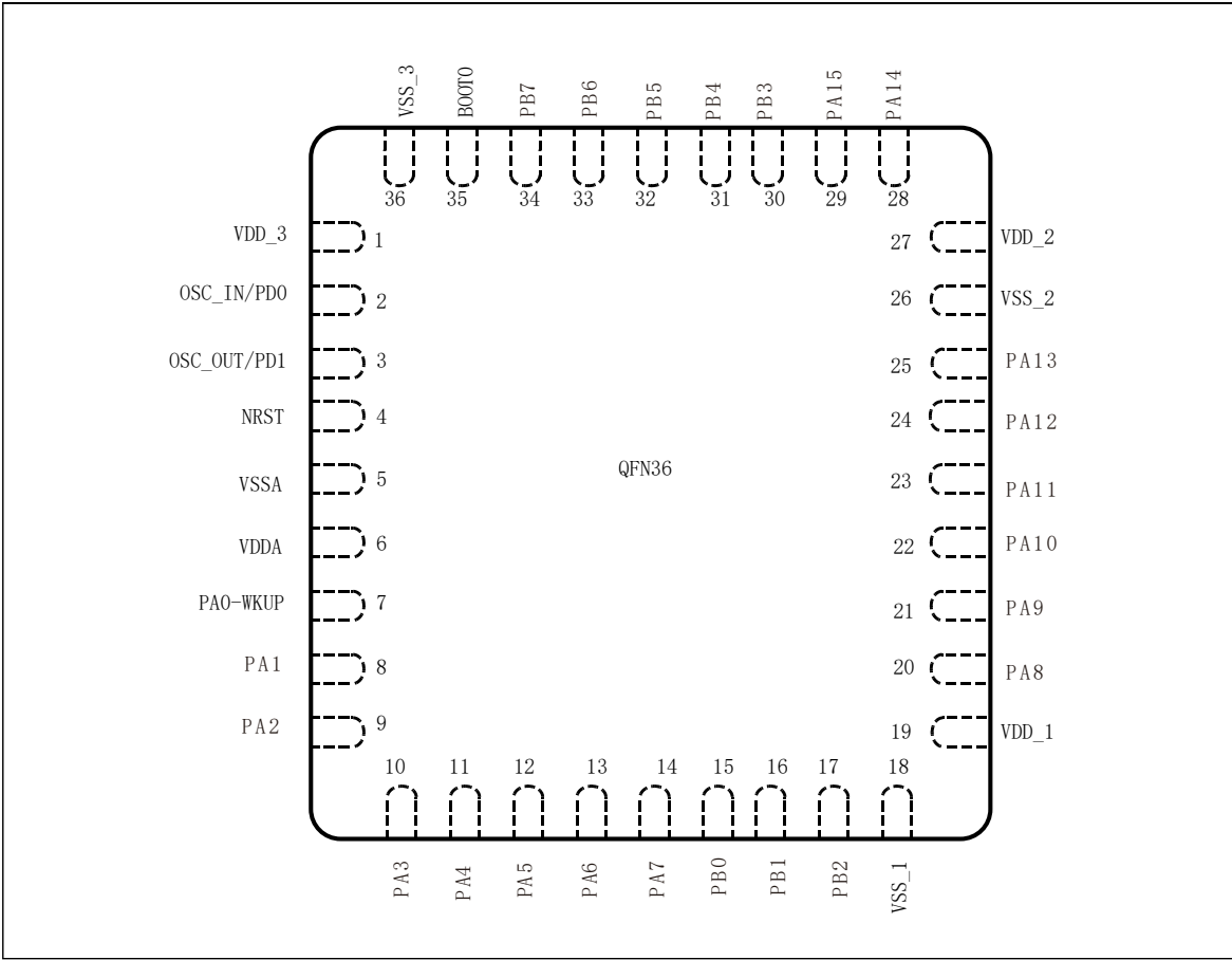
图 5-6 QFN36 引脚分布
