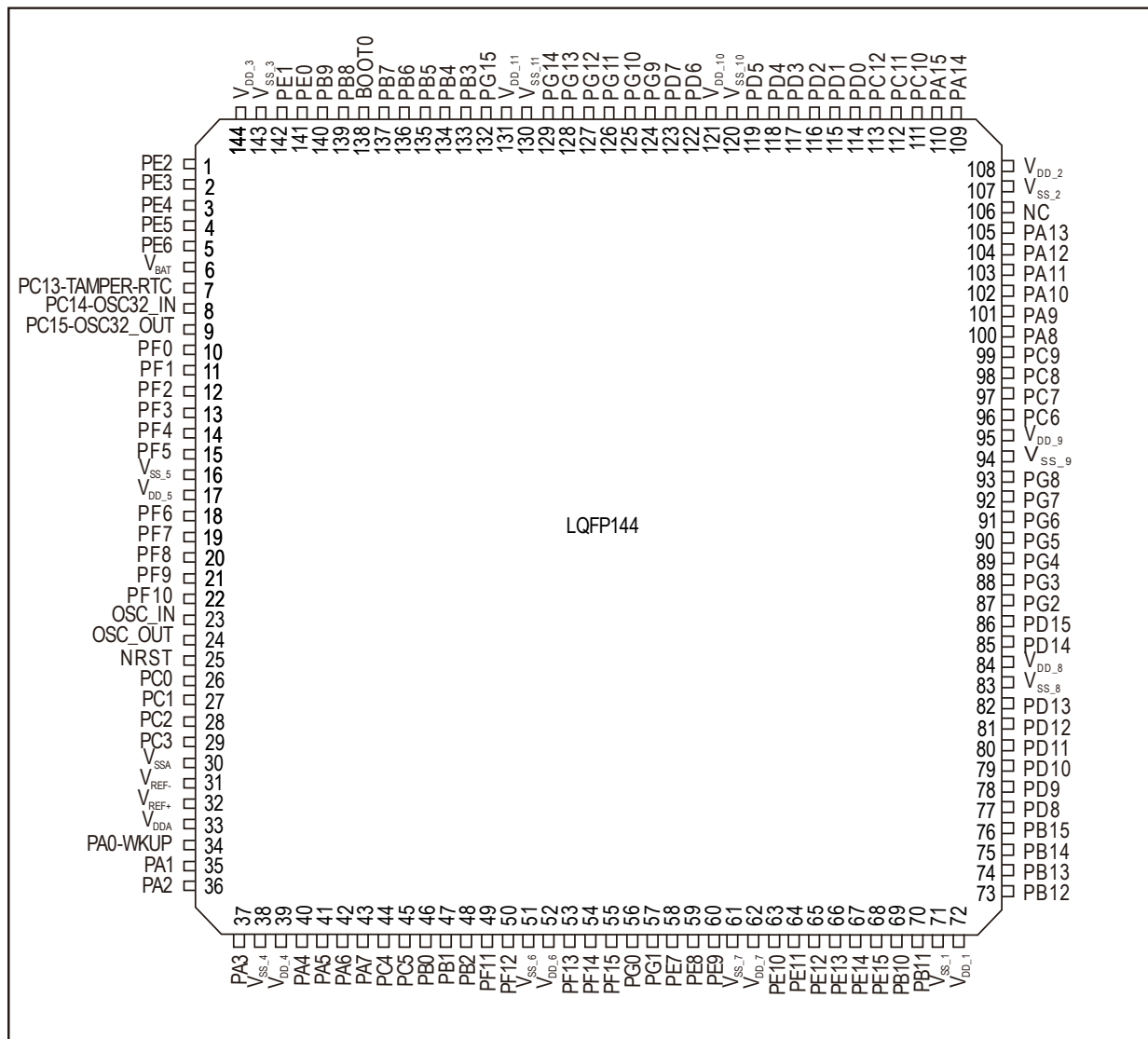
图 5-1 LQFP144 引脚分布
