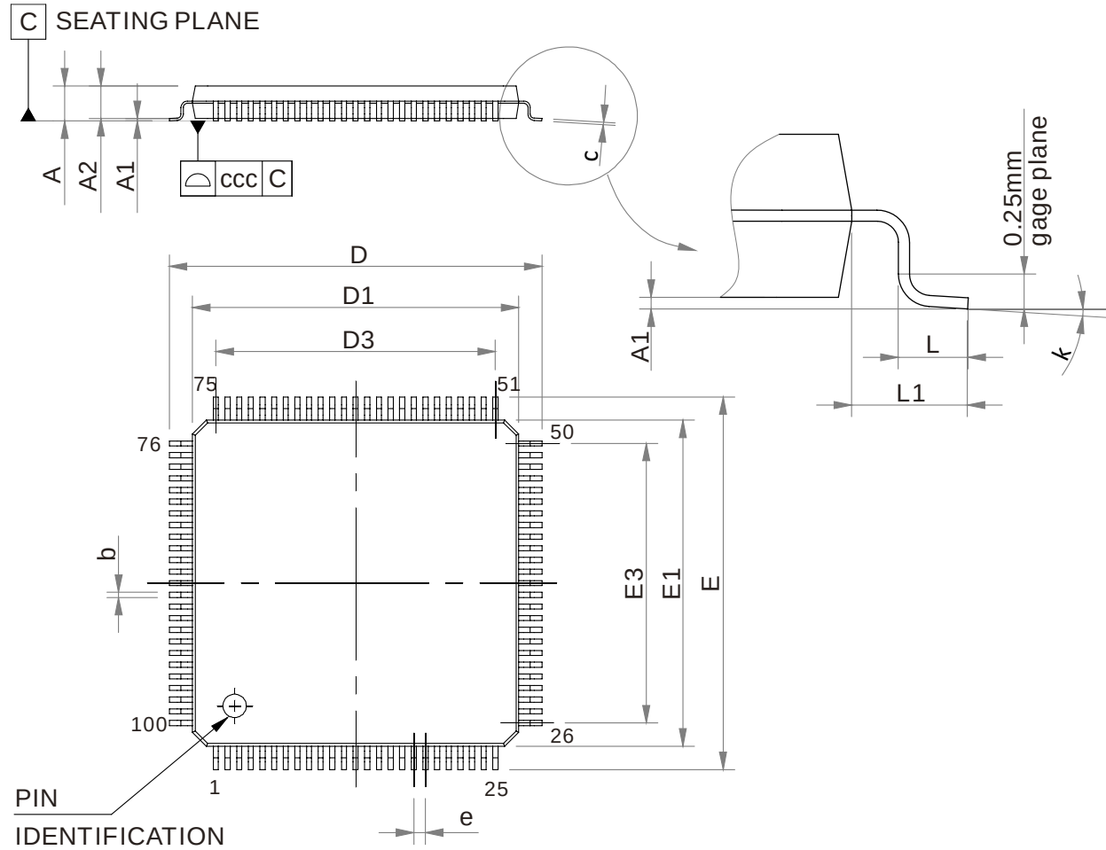
图 6-3 LQFP100 封装图
