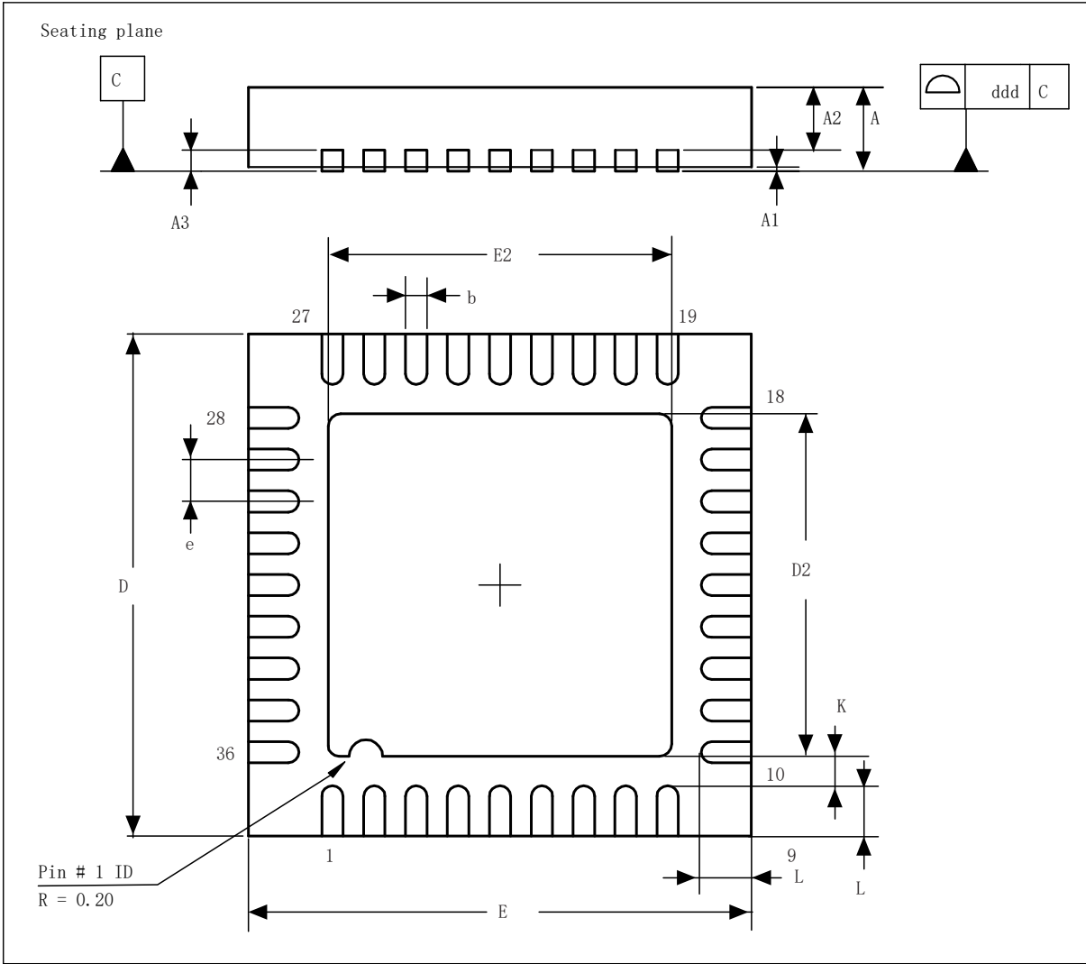
图 6-11 QFN36 封装图
